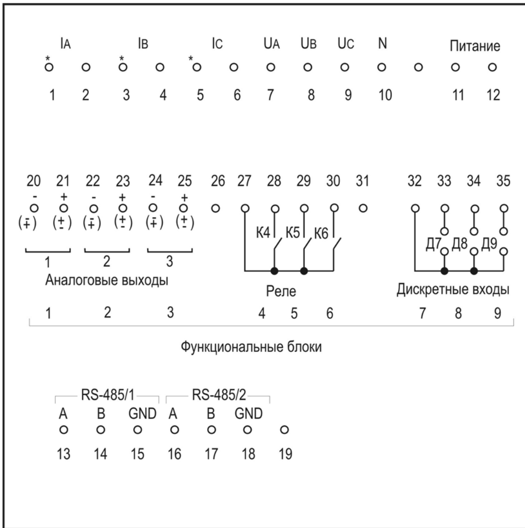
Рисунок В.3 - Схема подключения приборов, содержащих ОУ
