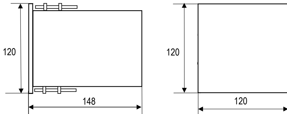
Рисунок 1 – Габаритные размеры ЦП 9010У
