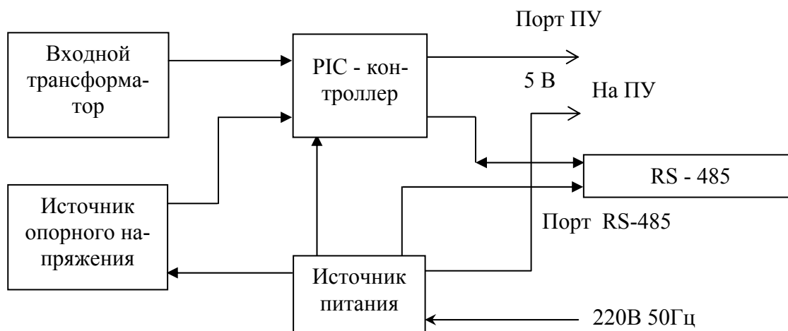
Рисунок 1 - Структурная схема прибора
