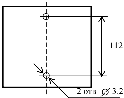
Рисунок Б.1 – Габаритные размеры ИП
