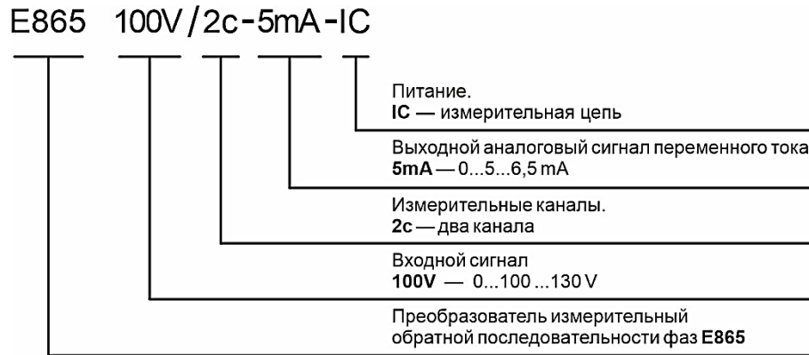
Рисунок 1 – Схема условного обозначения ИП переменного тока
