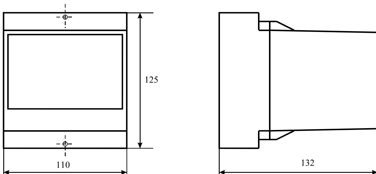
Рисунок Б.1 - Габаритные размеры ИП
