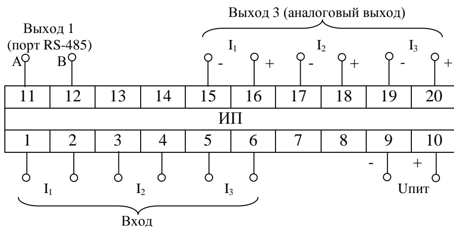
Рисунок А.1 - Схема электрическая подключений ИП
