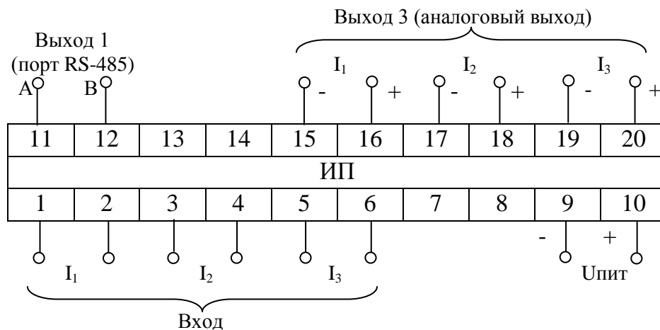
Рисунок Б.1 - Схема электрическая подключений ИП
