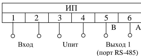
Рисунок Б.3 - Схема электрическая подключений ИП Е 854/2ЭС-ЦМ
