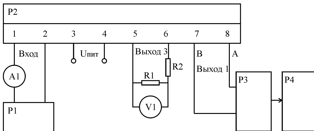
Рисунок А.3 – Схема проверки ИП Е 854/2ЭС-ЦМ
