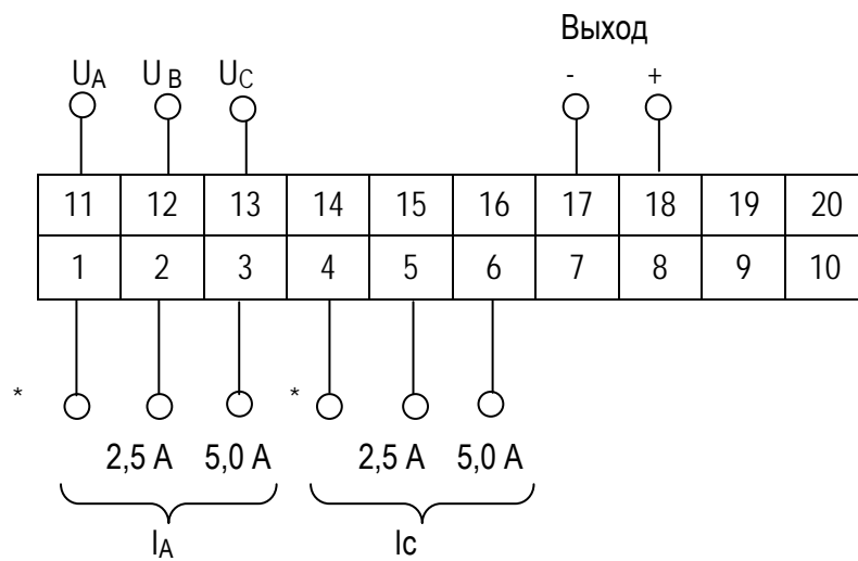
Рисунок А.3 – Схема подключения ИП Е 860/1ЭС, Е 860/3ЭС, Е 860/6ЭС, Е 860/8ЭС, Е 860/9ЭС
