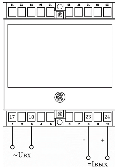
Рисунок Б.1 – Схемы электрические подключения ИП в корпусе E20
