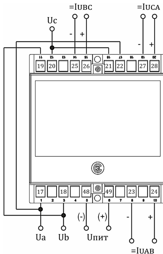
б) Корпус Е20 (3 входа, 3 аналоговых выхода) схема для контроля междупазных напряжений
