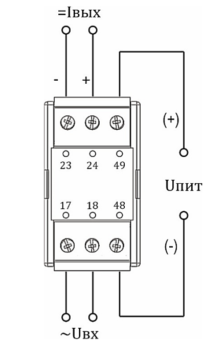
а) Корпус М6 (1 вход, 1 аналоговый выход)
