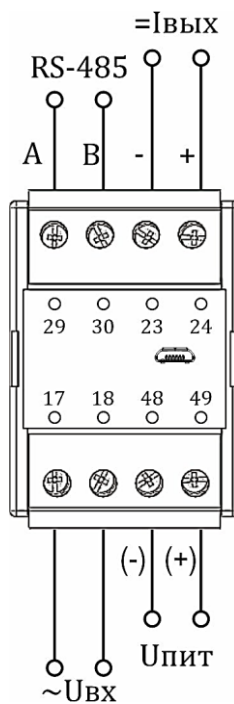
в) Корпус М8 (1 вход, 1 аналоговый выход, 1 порт RS-485, 1 порт USB)
