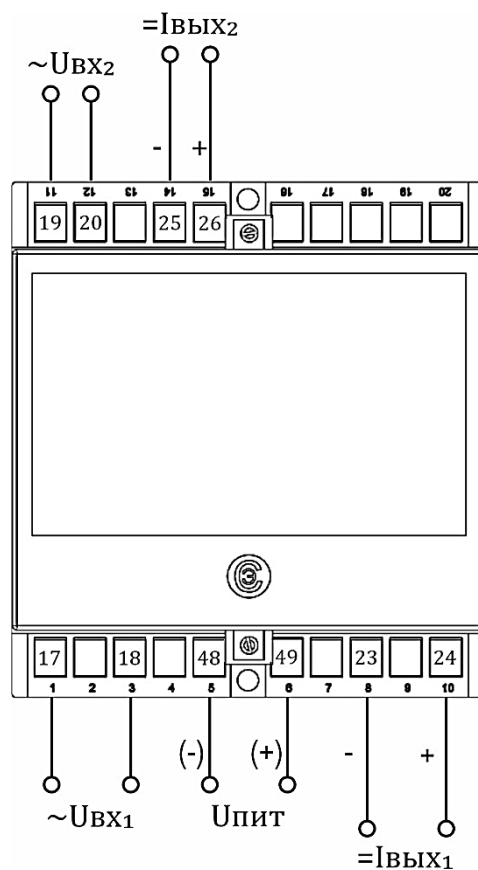
б) Корпус Е20 (2 входа, 2 аналоговых выхода)
