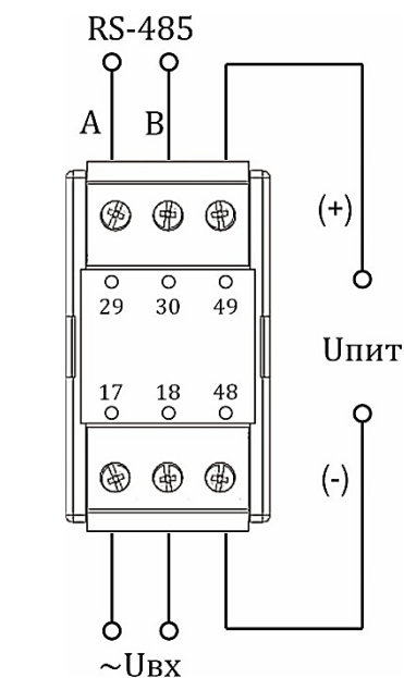
б) Корпус М6 (1 вход, 1 порт RS-485)
