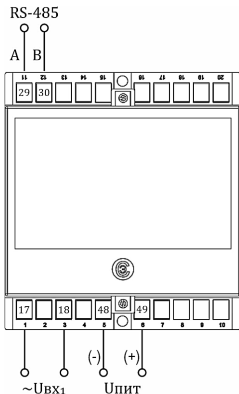
а) Корпус E20 (1 вход, 1 порт RS-485)
