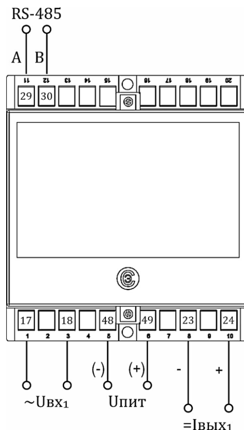
б) Корпус E20 (1 вход, 1 аналоговый выход, 1 порт RS-485)
