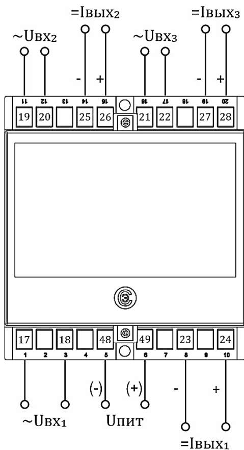
а) Корпус Е20 (3 входа, 3 аналоговых выхода) схема для контроля фазных напряжений
