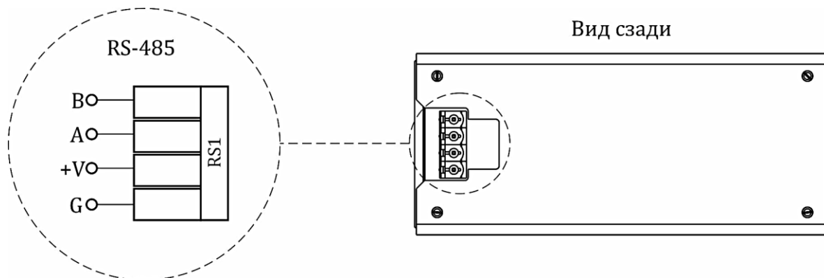
Рисунок Б.7 – Схемы электрические подключения E8DU
