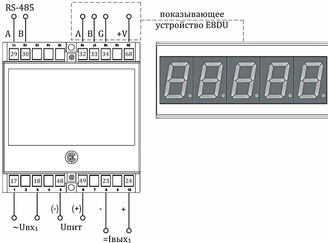
Корпус EB20 (ИП, содержащие порт показывающего устройства)
