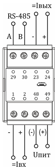
Корпус М8 (1 вход, 1 аналоговый выход, 1 порт RS-485)
