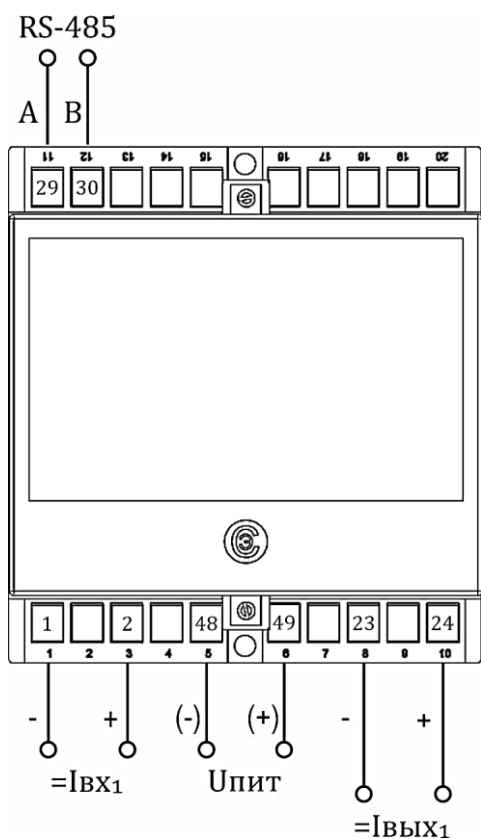
а) Корпус E20 (1 вход, 1 аналоговый выход, 1 порт RS-485)
