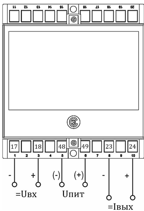
а) Корпус E20 (1 вход, 1 аналоговый выход)
